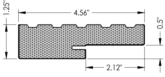
2 COMPOSITE JAMB
