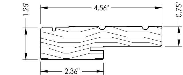
1 WOOD JAMB
